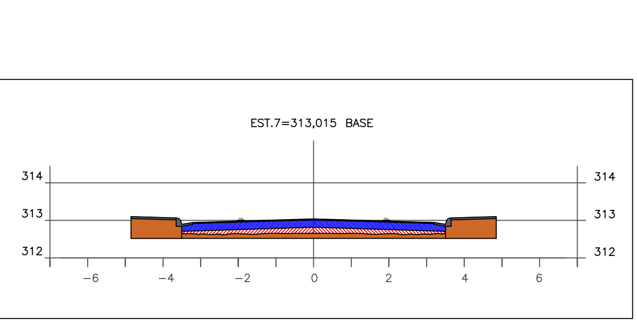
SEÇÕES DO PAVIMENTO ESCALA 1/100
