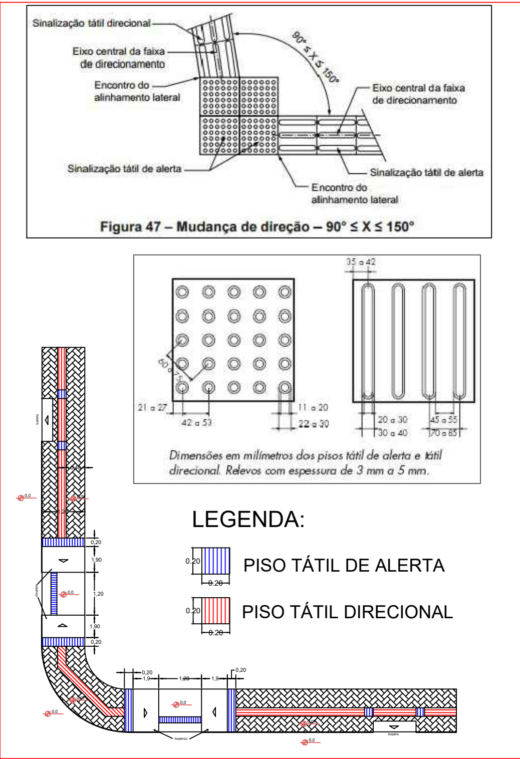
DETALHE - PISOS TÁTEIS ESCALA S/E
