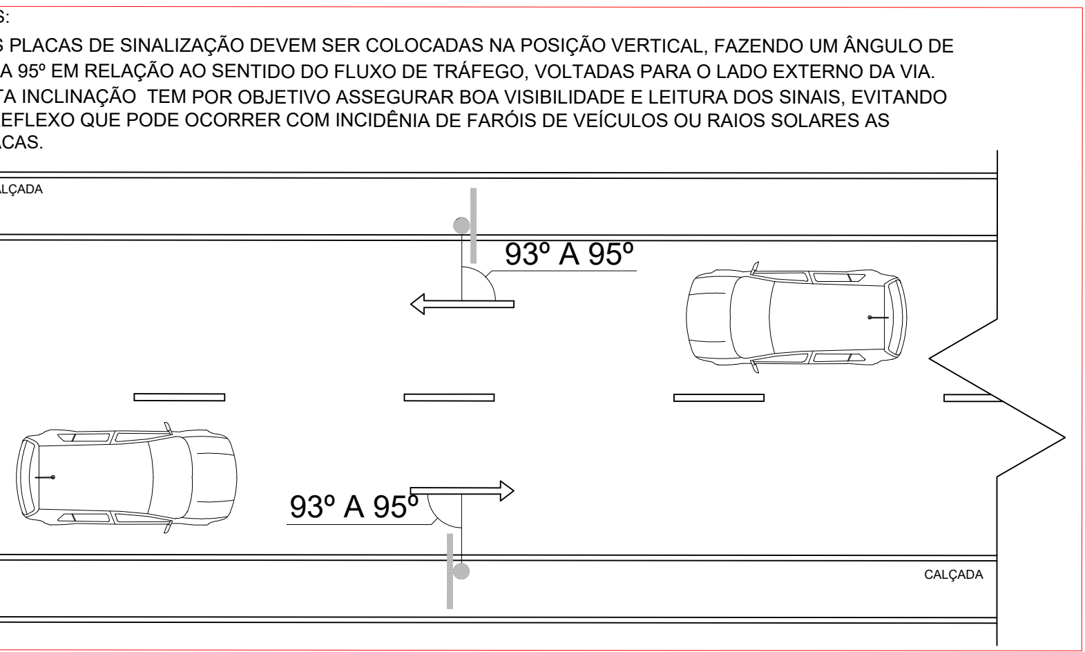
DETALHE - LOCAÇÕES DE PLACAS ESCALA S/E
