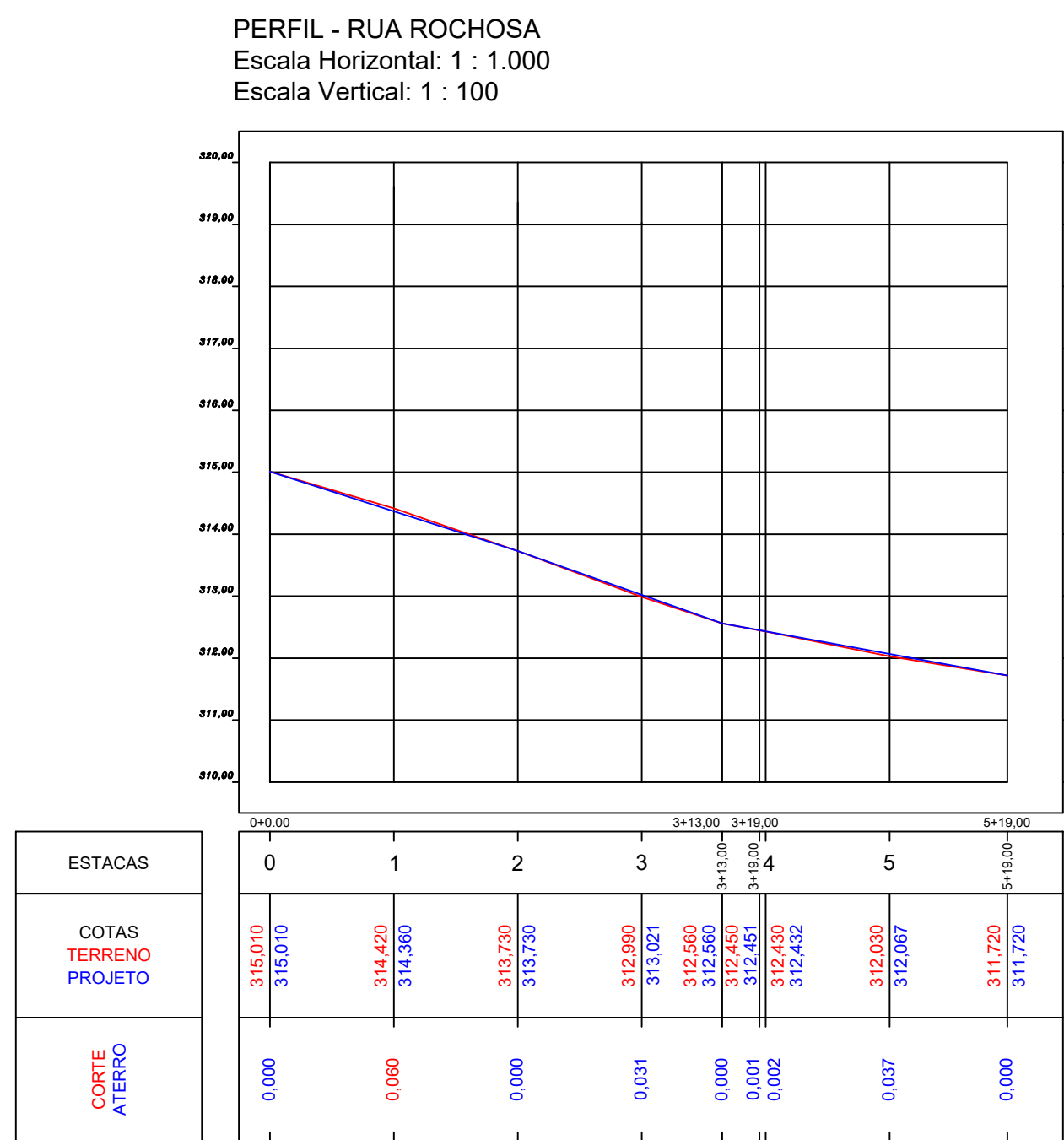
PERFIL LONGITUDINAL ESCALA H. 1/1000 ESCALA V. 1/100
