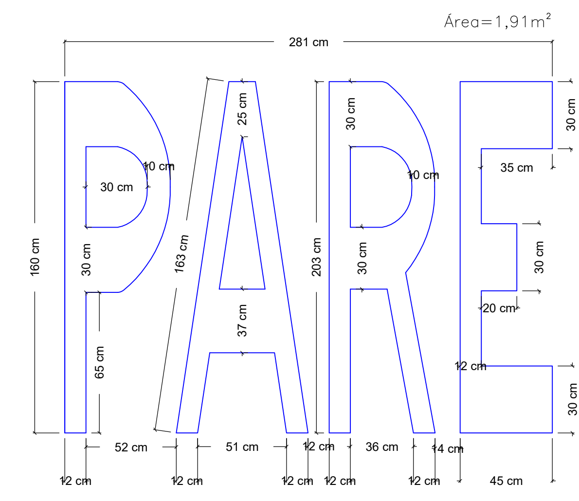
DETALHE - SINALIZAÇÃO DE PARADA OBRIGATORIA ESCALA S/E
