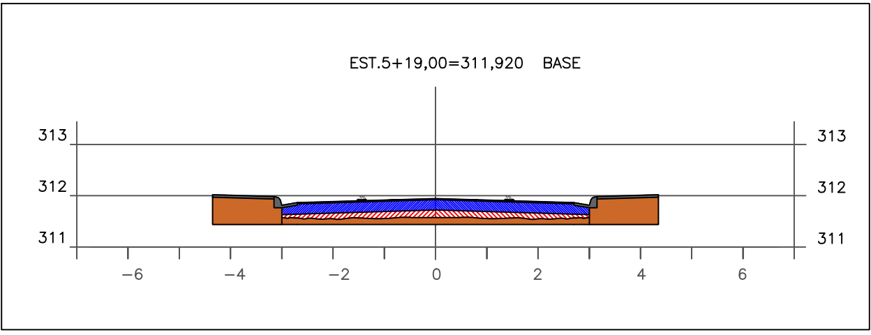
SEÇÕES DO PAVIMENTO ESCALA 1/100
