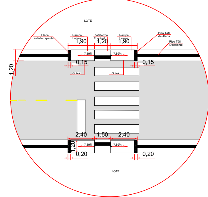
DETALHE - CALÇADAS E RAMPAS ESCALA S/E
