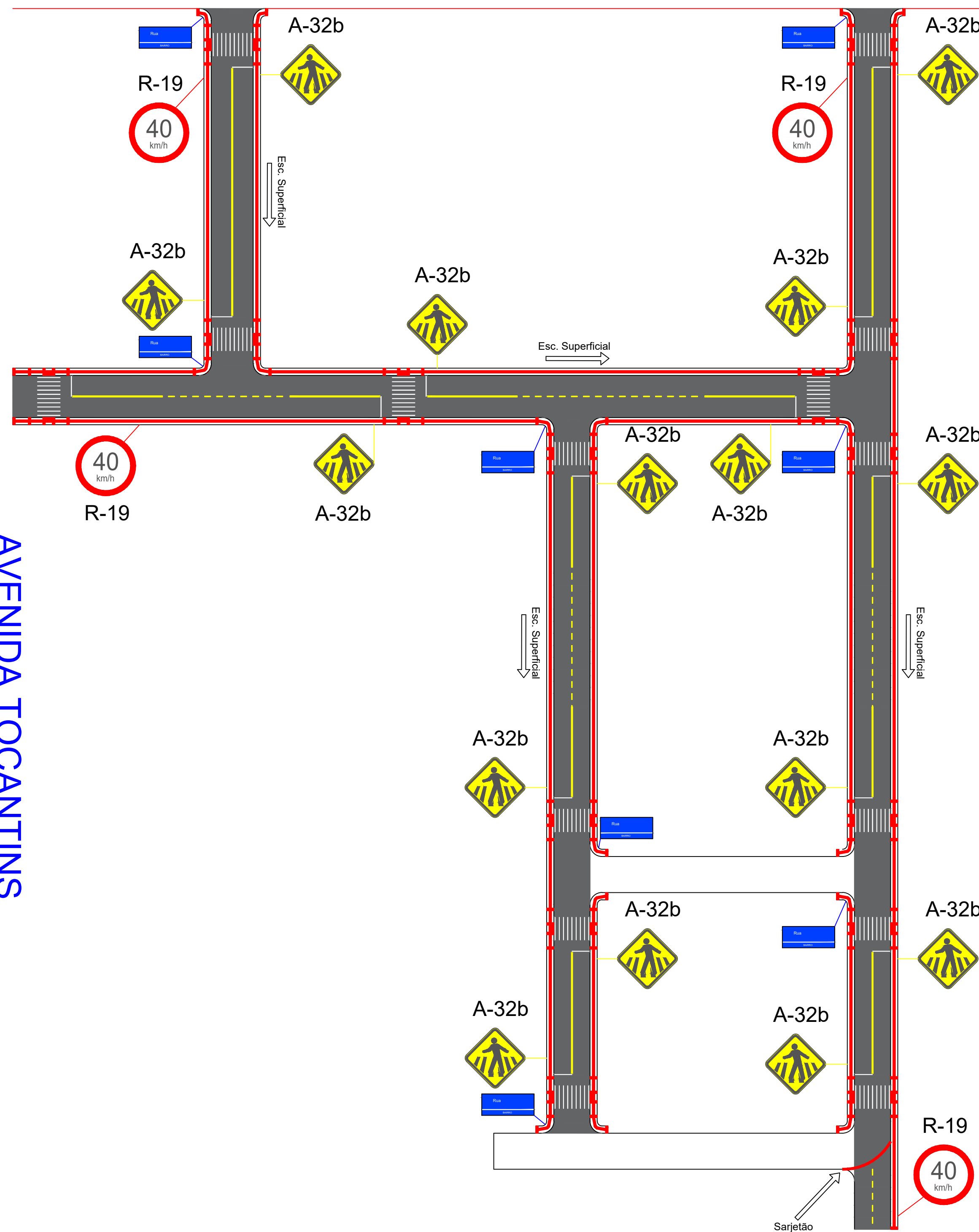
PLANTA DE IMPLANTAÇÃO ESCALA 1/500
