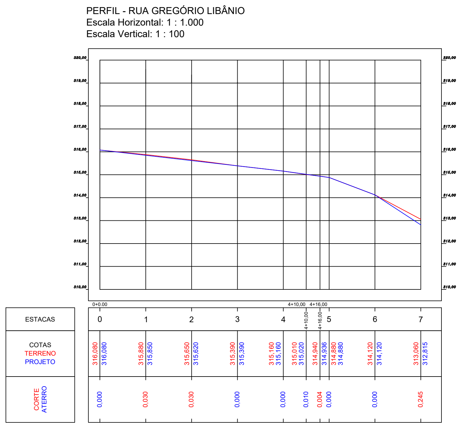
PERFIL LONGITUDINAL ESCALA H. 1/1000 ESCALA V. 1/100
