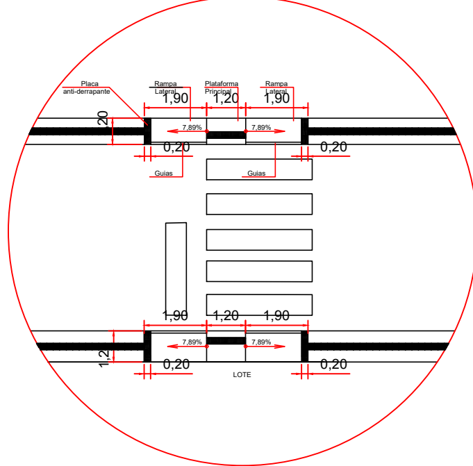
DETALHE - CALÇADAS E RAMPAS ESCALA S/E
