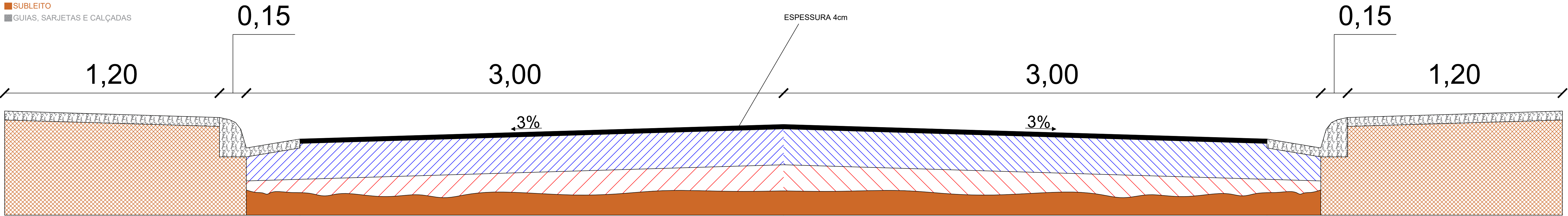
SEÇÃO TIPO - PAVIMENTO ESCALA 1/10
