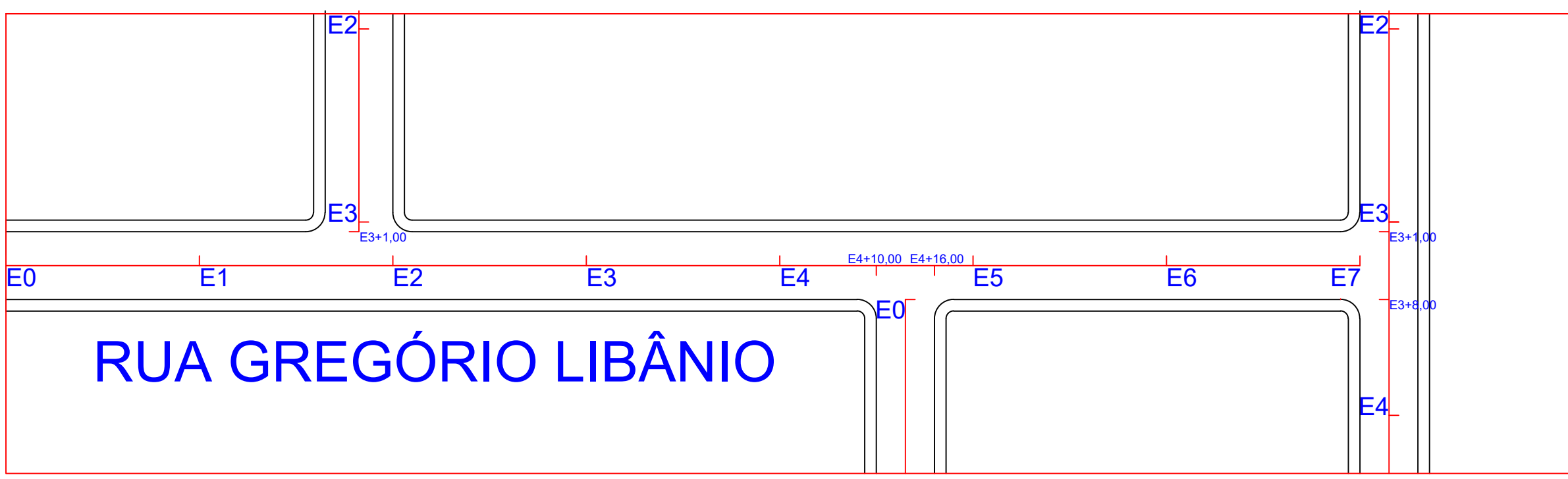
PLANTA DE LOCAÇÃO ESCALA 1/500
