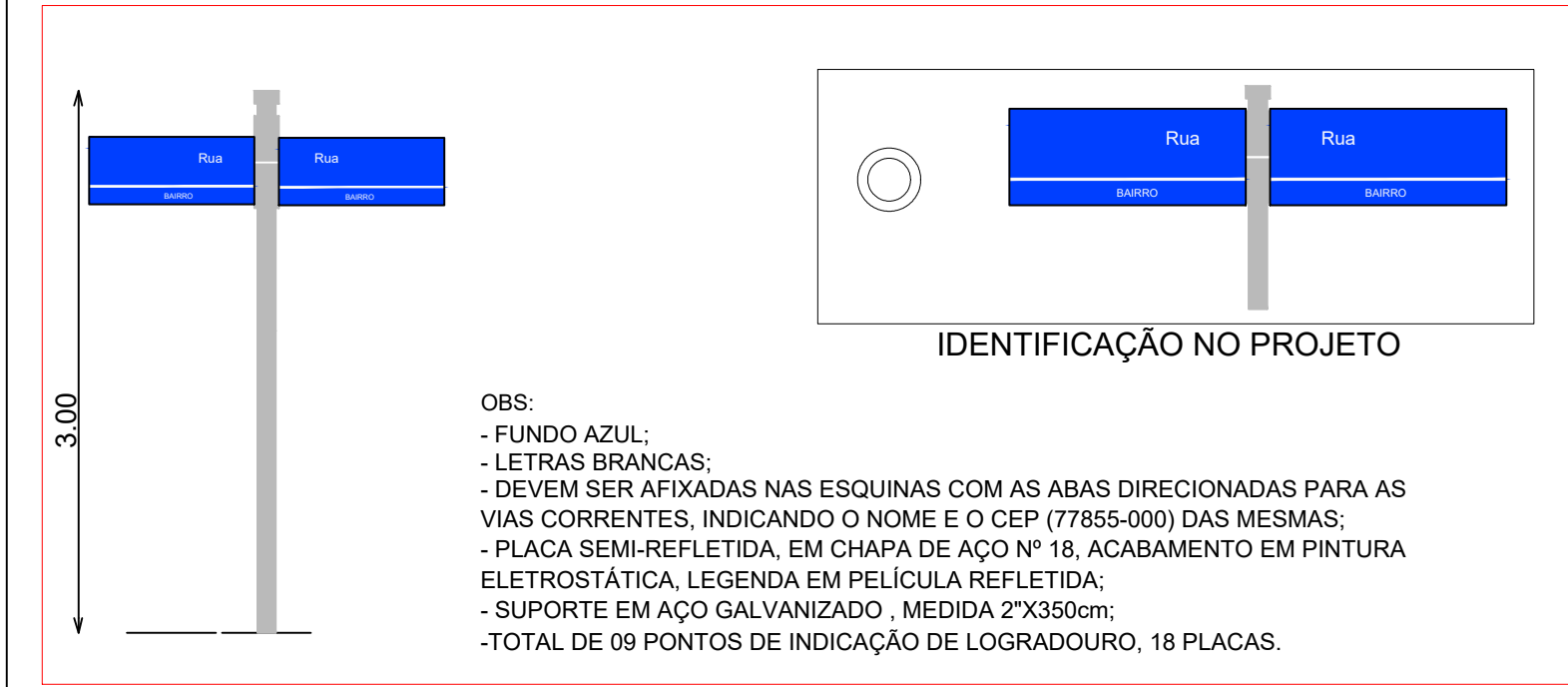
DETALHE - SINALIZAÇÃO DE IDENTIFICAÇÃO DE LOGRADOURO ESCALA S/E
