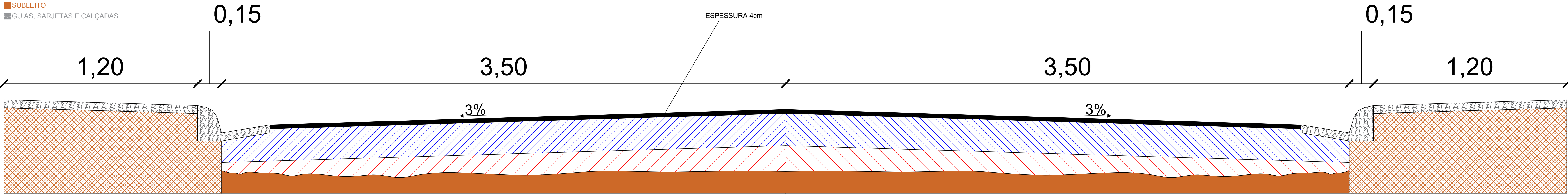
SEÇÃO TIPO - PAVIMENTO ESCALA 1/10
