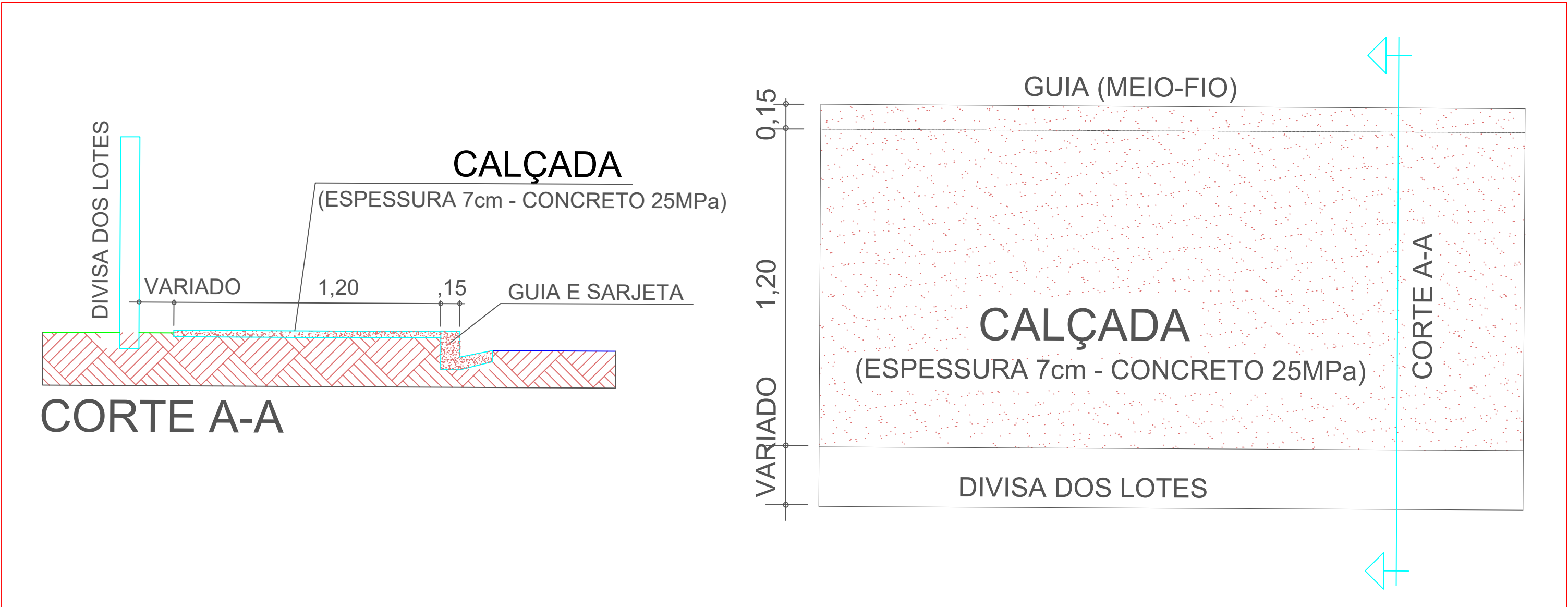
DETALHE - CALÇADAS ESCALA S/E
