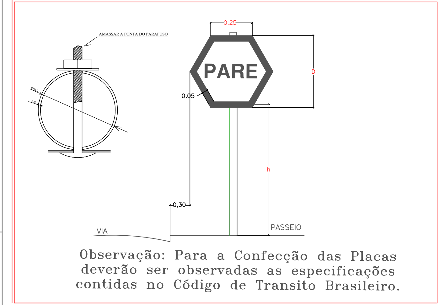
DETALHE - LOCAÇÕES DE PLACAS ESCALA S/E
