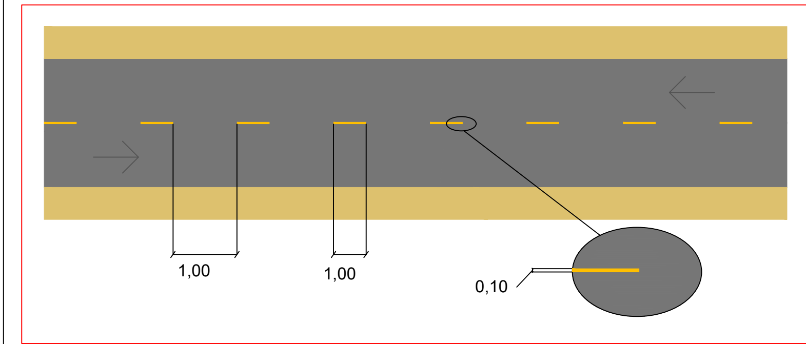
DETALHE - FAIXA AMARELA SECCIONADA ESCALA S/E
