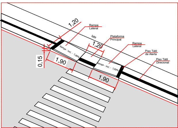
DETALHE - CALÇADAS E RAMPAS ESCALA S/E
