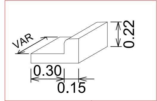
DETALHE - GUIAS E CALÇADAS ESCALA S/E
