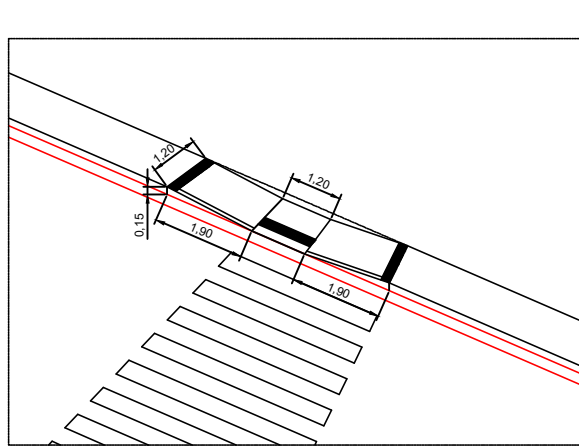
DETALHE - RAMPAS ESCALA S/E
