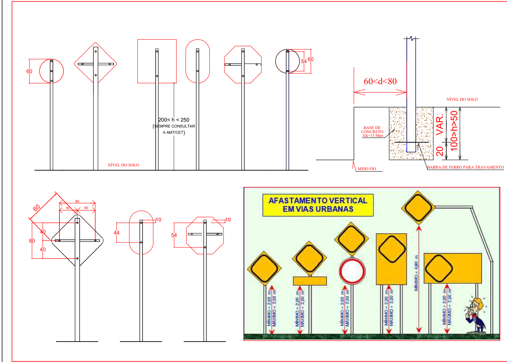
DETALHE - SINALIZAÇÃO VERTICAL ESCALA S/E
