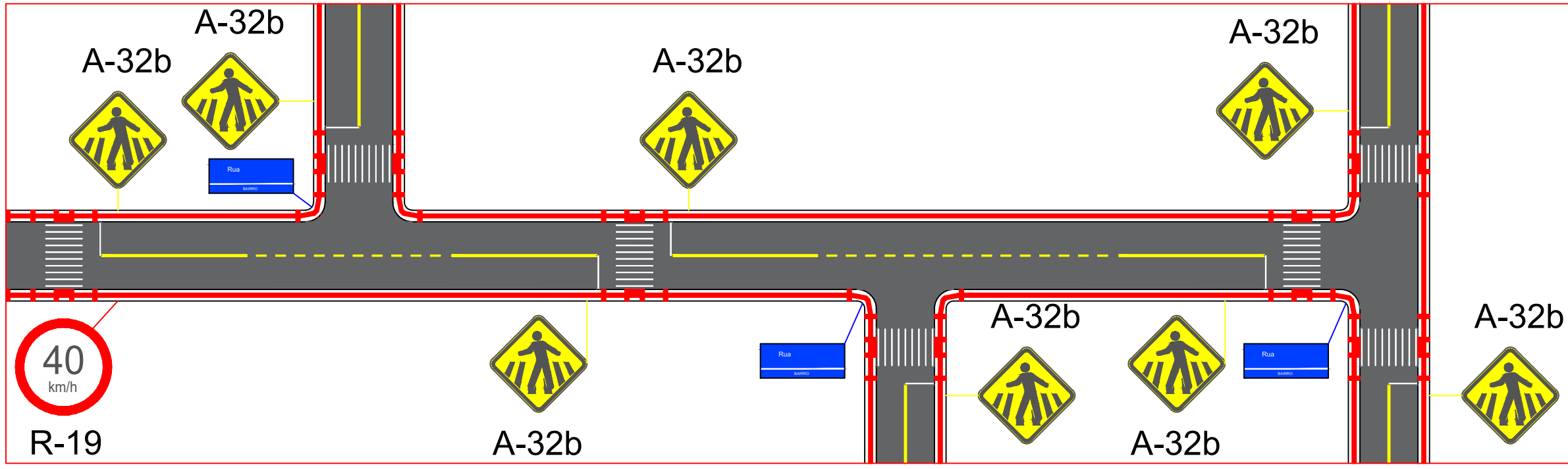
PLANTA DE IMPLANTAÇÃO ESCALA 1/500
