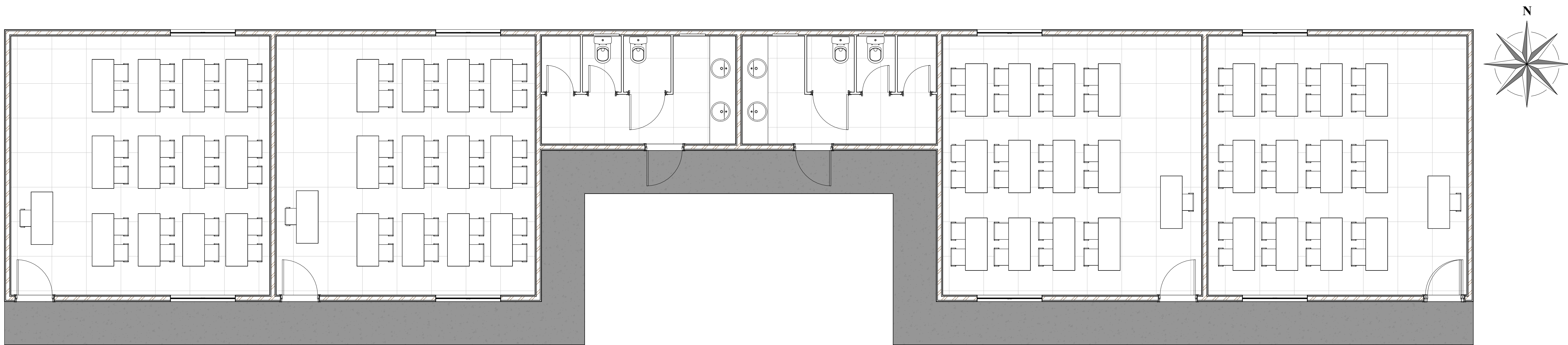
2 PLANTA DE LAYOUT 1 : 50
