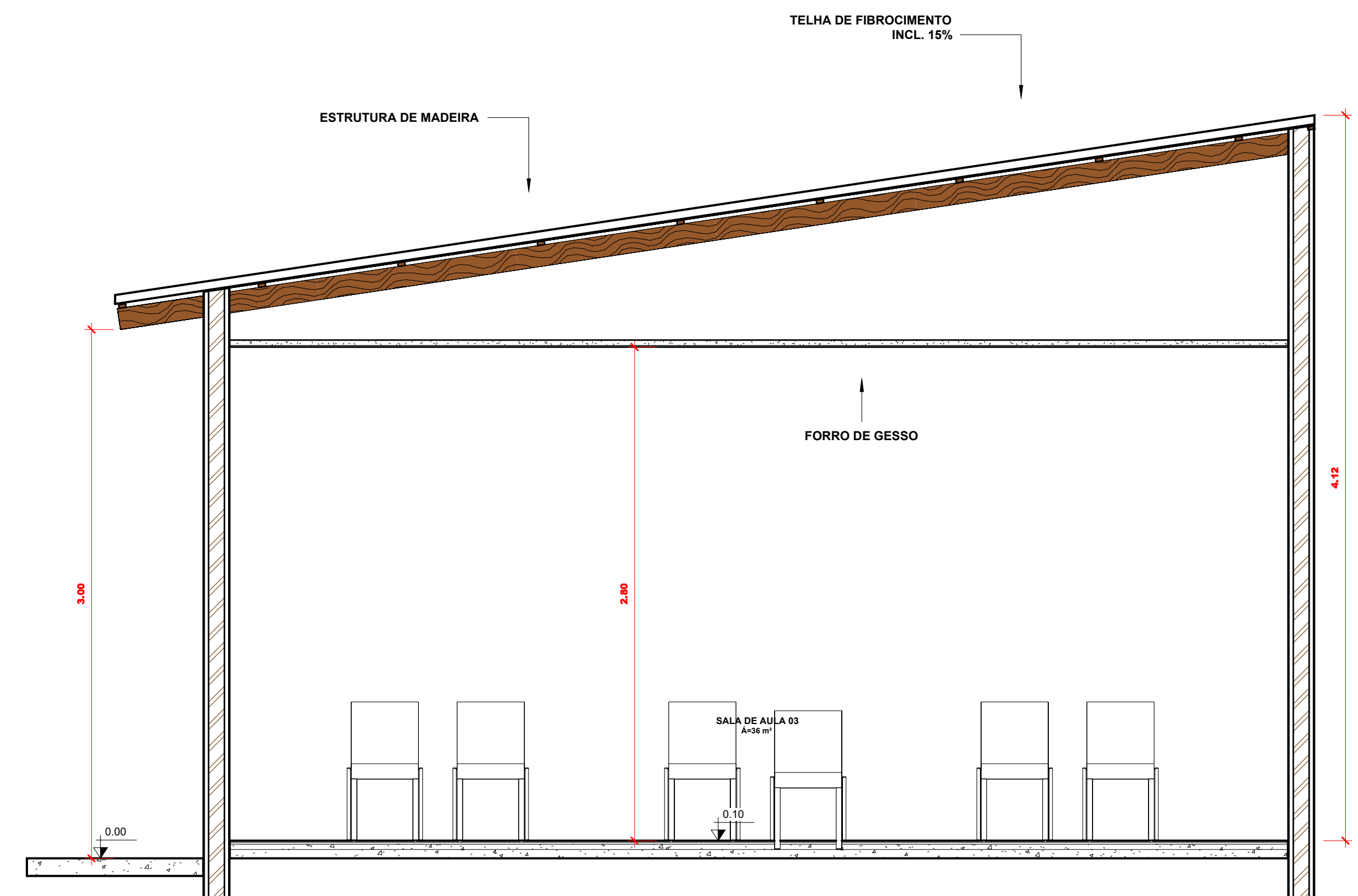
4 Corte AA 1 : 25
