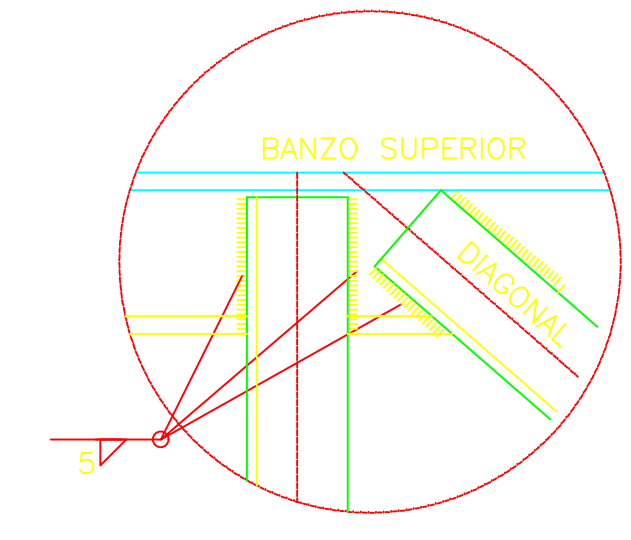
DETALHE 02 ESCALA: 1:5
