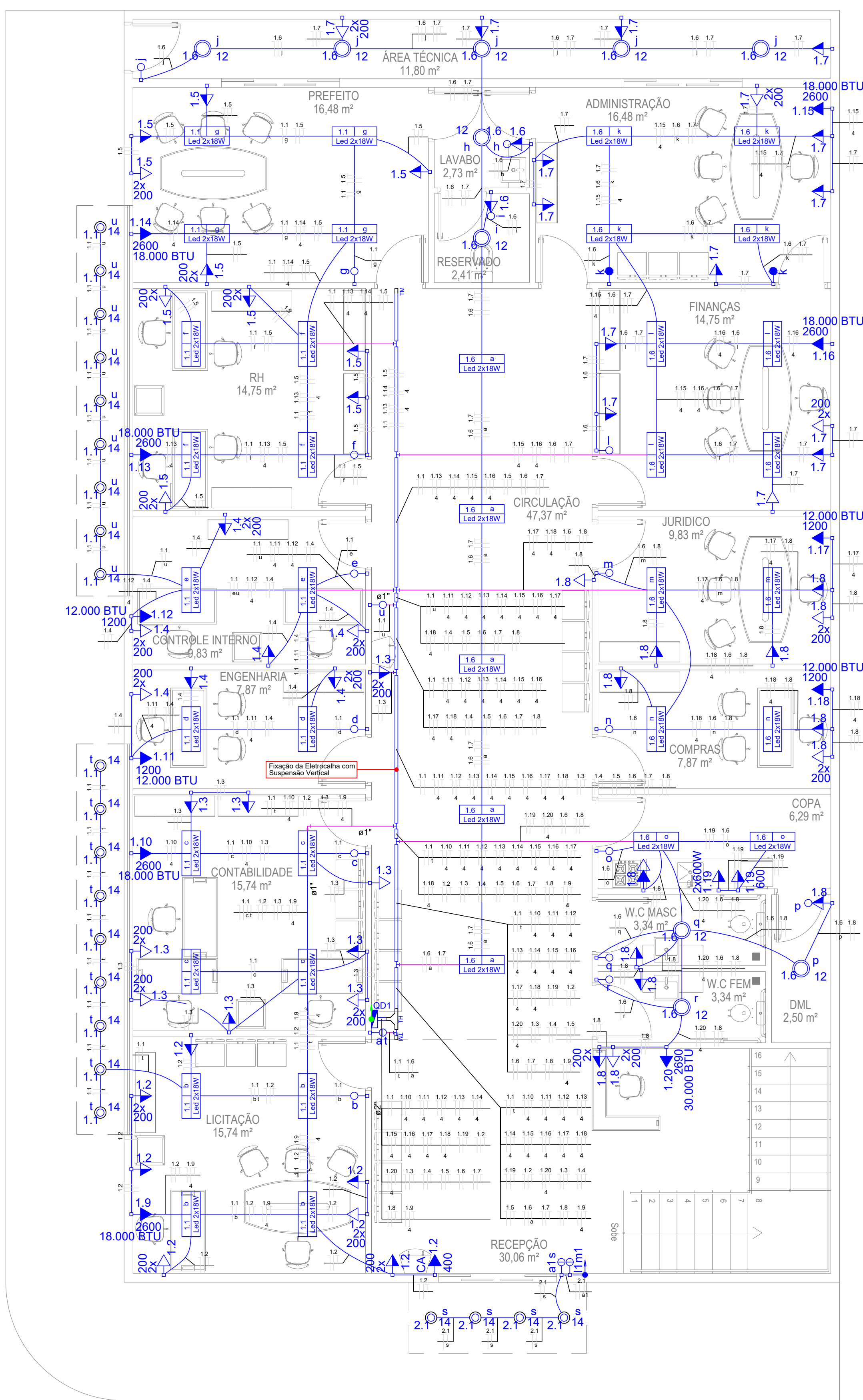
PLANTA ELÉTRICA - TÉRREO Escala 1/50
