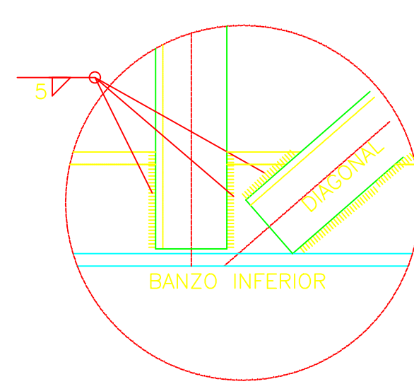
DETALHE 03 ESCALA: 1:5
