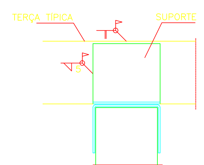
DETALHE 01 ESCALA: 1:5
