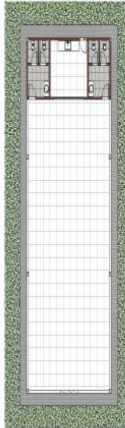
② Planta de Layout - Térreo 1:100
